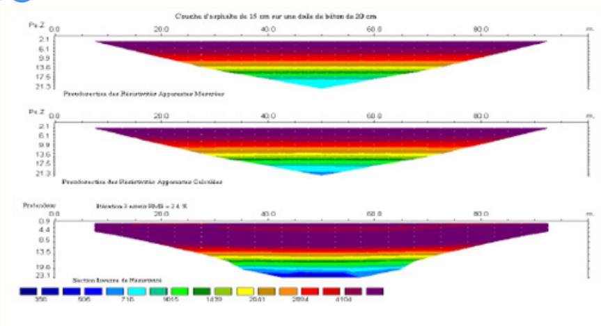
Sondage électrique et Tomographie électrique
