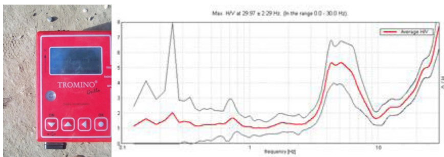
Tromino et enregistrement passif
