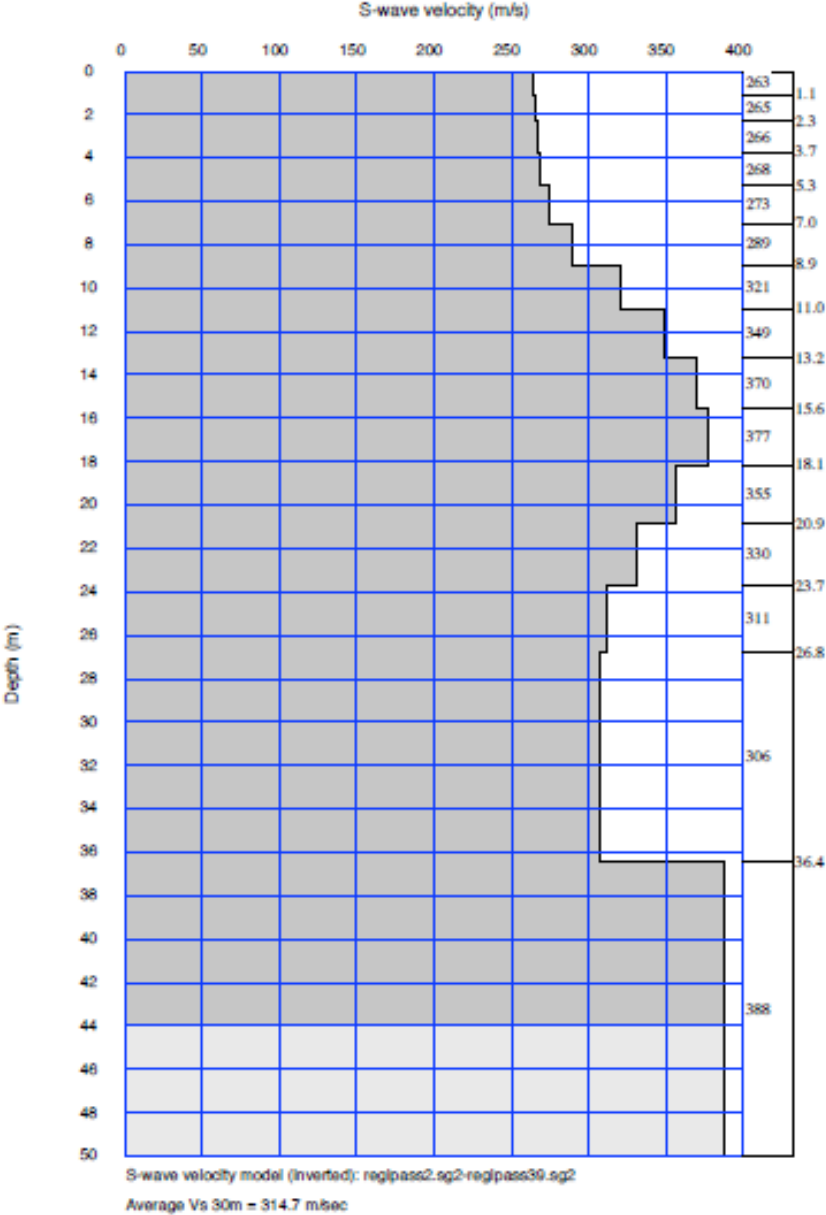
Exemple de profil V_{s30}
