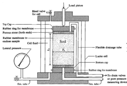
(a) Schéma de principe d'une cellule triaxiale (d'après Bowles, 1995).
