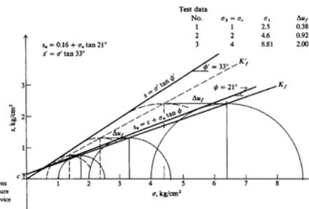
(b) Exemple de courbe intrinsèque construite à partir de trois essais triaxiaux ; critère de Mohr-Coulomb (ibidem).
