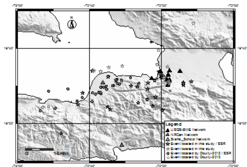
Localisation des stations sismiques de différents réseaux permanents. Les cercles pleins représentent les événements utilisés pour l'analyse SSR et les cercles vides pour les événements non enregistrés dans la station de référence ou trop proches des stations d'enregistrement. ST Fleur et al., In prep
