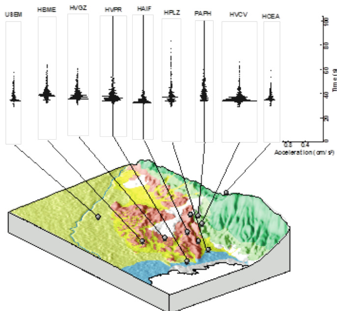
Bloc diagramme montrant la distribution spatiale des accélérations sismiques dans la direction Nord-Sud pour la Réplique du 3 mai 2010 ( M_w=4.4 ), ST Fleur et al., In prep.
