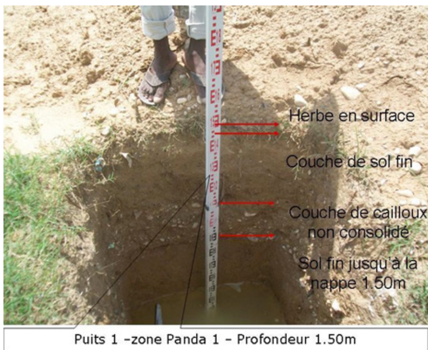
Exemple de puits manuel
